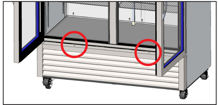
Рис. 1. Виты крепления жалюзийной решетки под распашными дверцами
