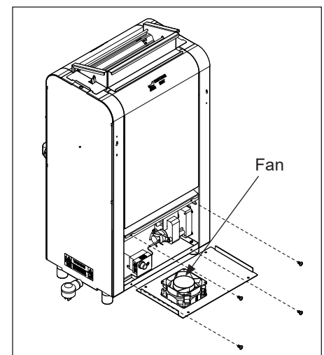
Figure 25. Rear fan
